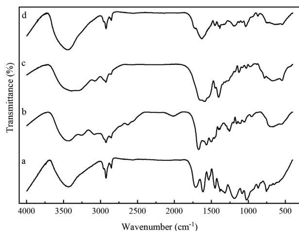
Fig. 1. FT-IR spectra: a) tannic acid; b) \epsilon -PL; c) \gamma -PGA; d) PGA-PL-tannin gel.
