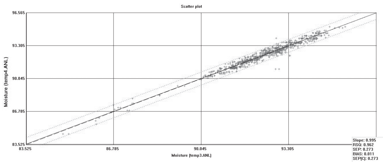
Fig. 8. Scatter plot moisture content press final effluent.
