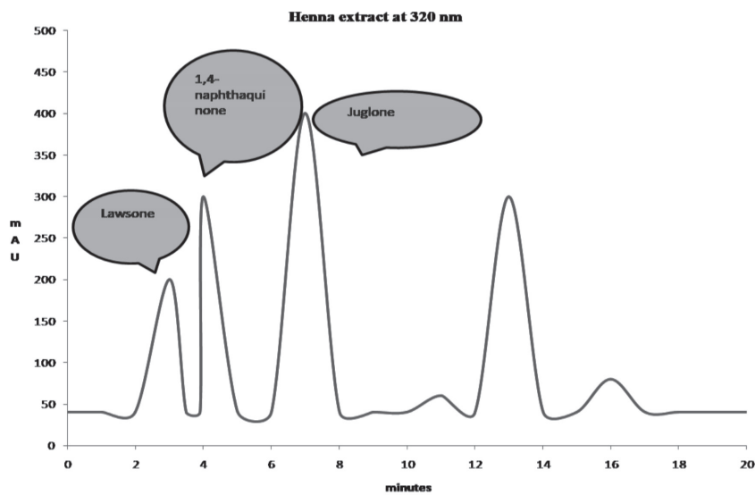
Fig. 4. HPLC-DADchromatogram of Lawsonia inermis L.
