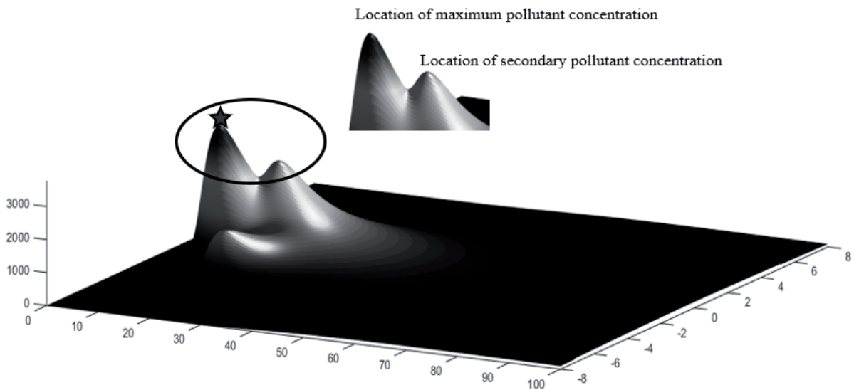
Fig. 5. Pollutant diffusion concentration map.
