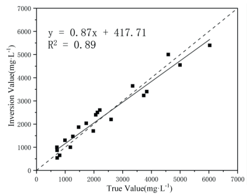
(f) BO-XGBoost
